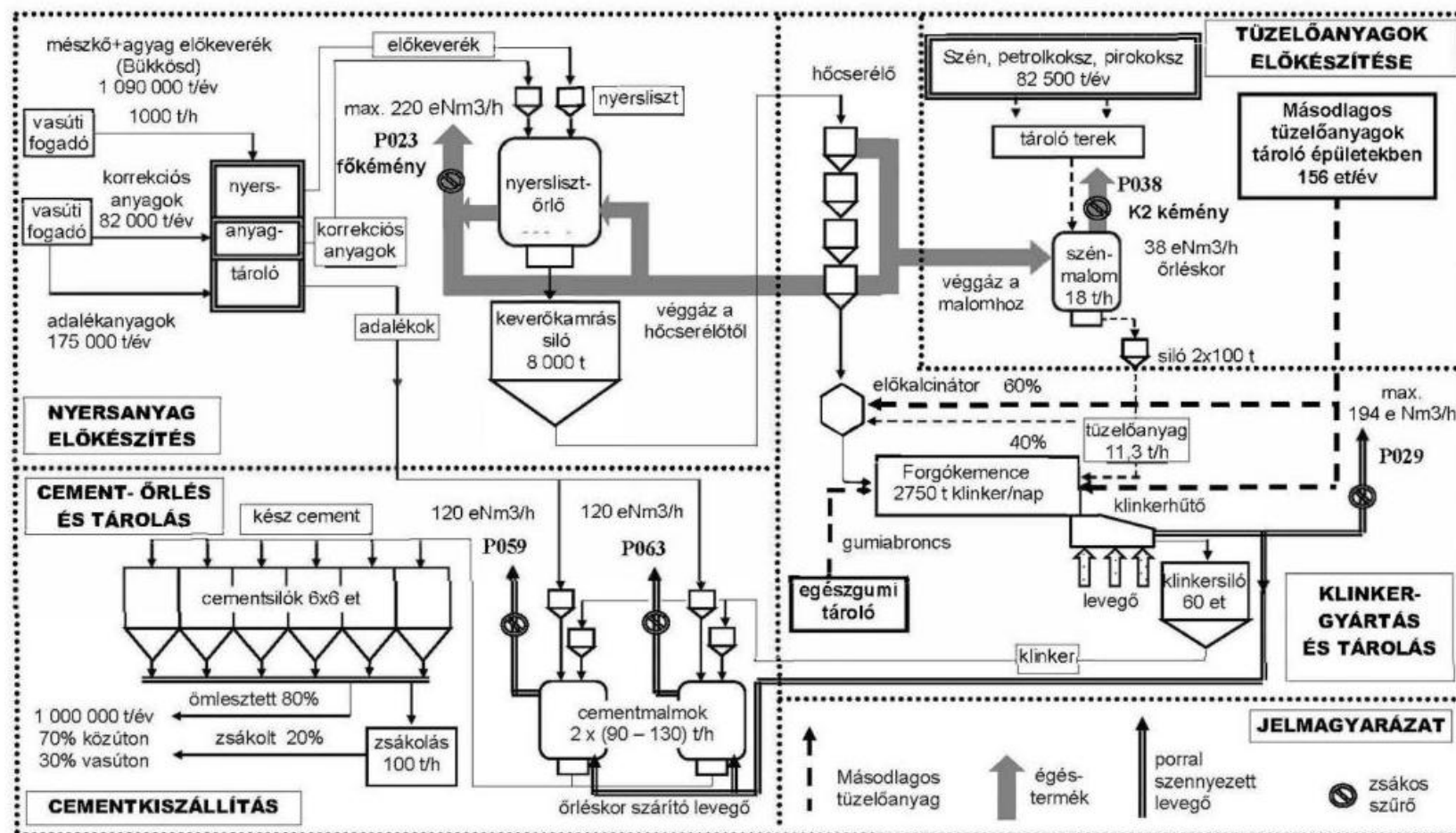
1. ábra Egyszerűsített technológiai folyamatábra
