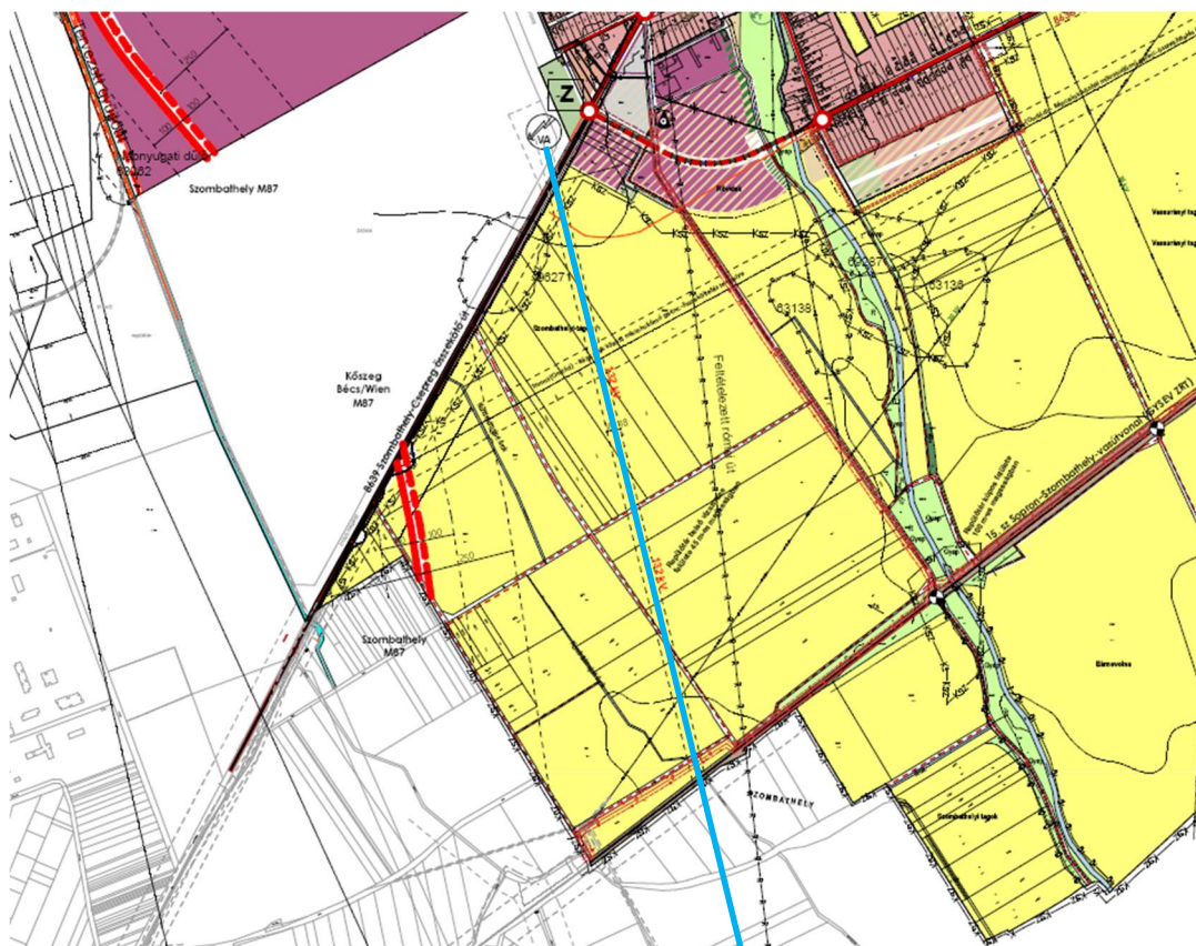
2. ábra – Söpte településszerkezeti terv részlete a tervezett nyomvonallal (kék vonal: 132 kV tervezett távvezeték)
