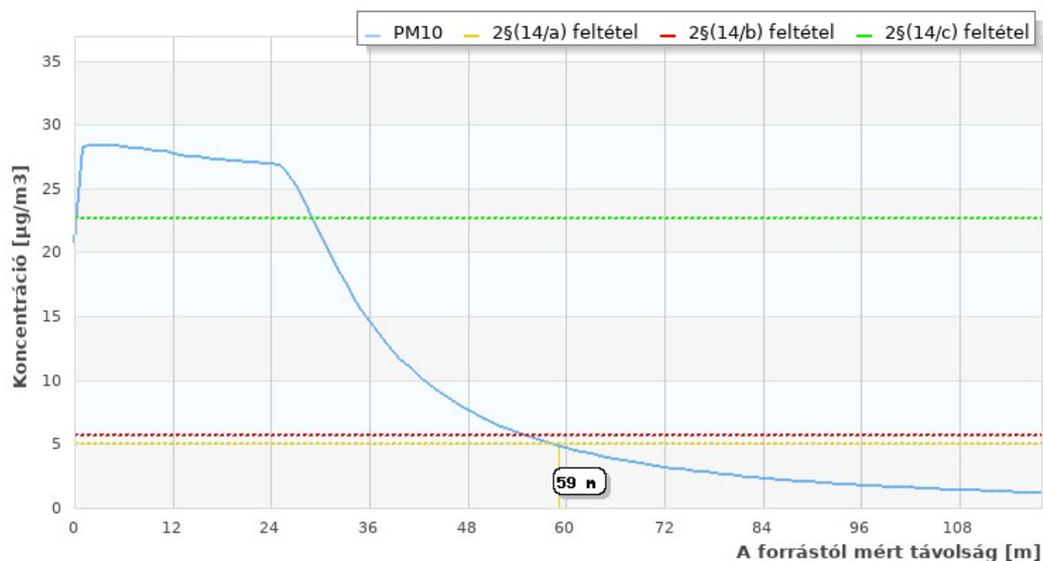
5. ábra – Munkaterület PM10 kibocsátásának 24 órás terjedésmodell görbéje
